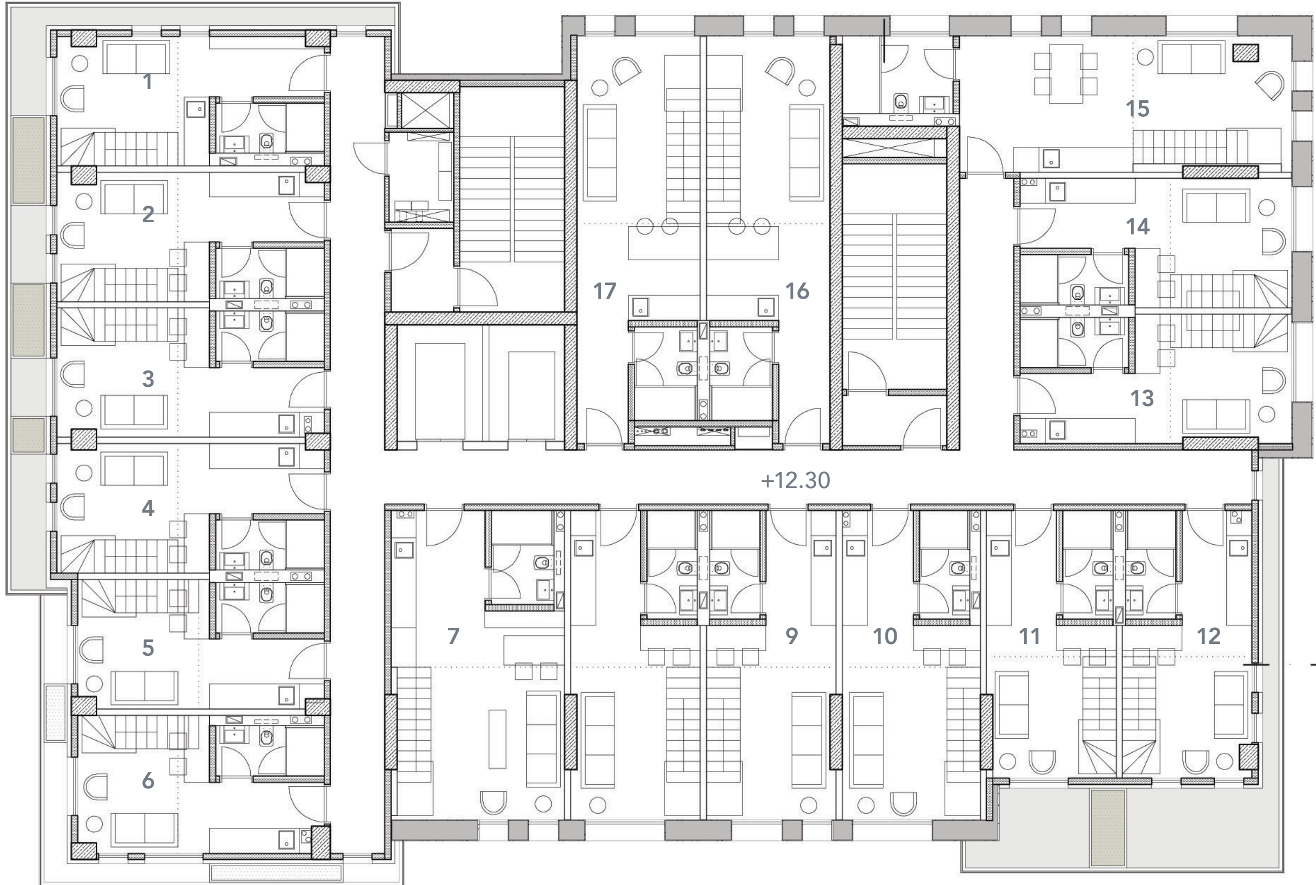
3. Kat Planı
