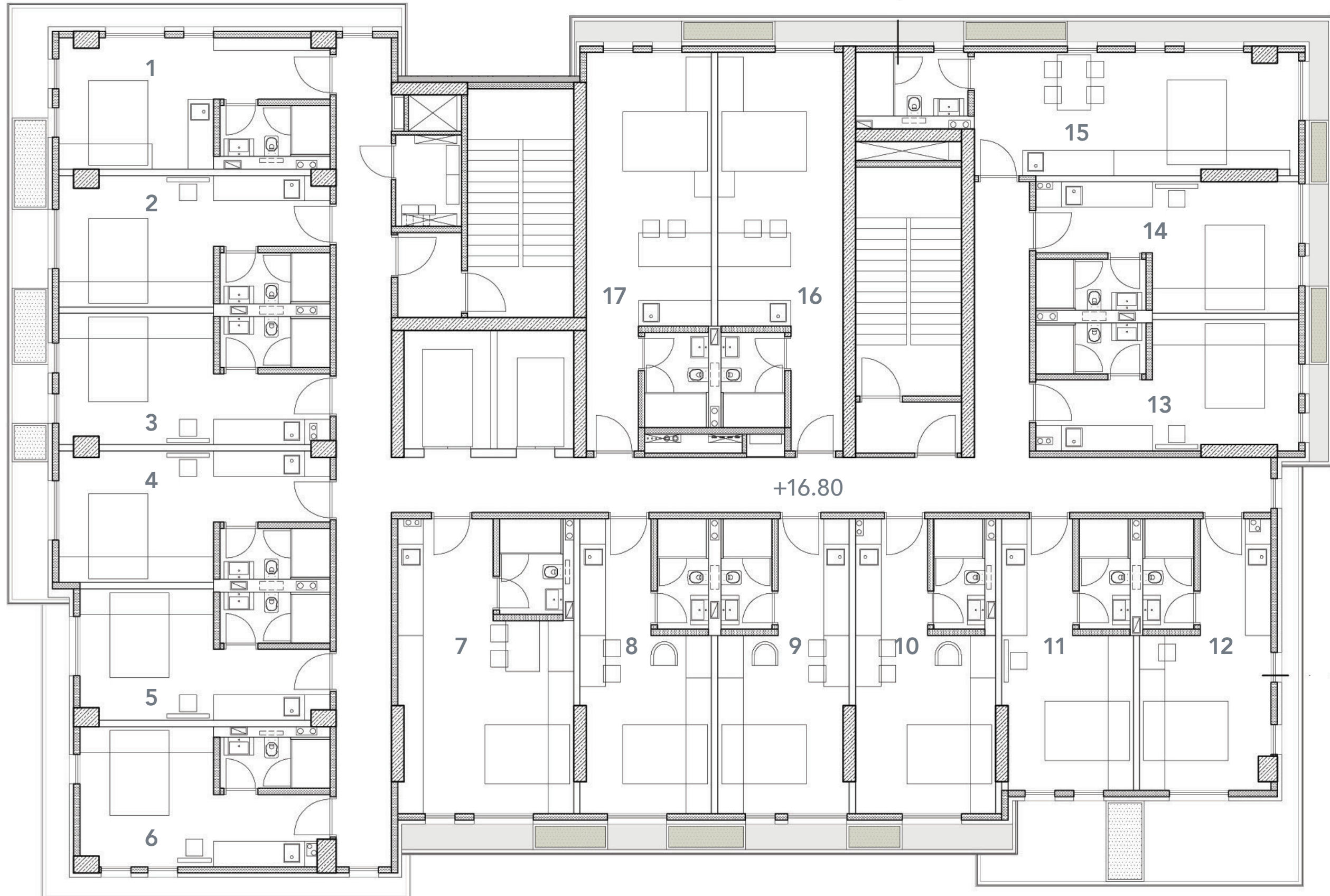
4.Kat Planı
